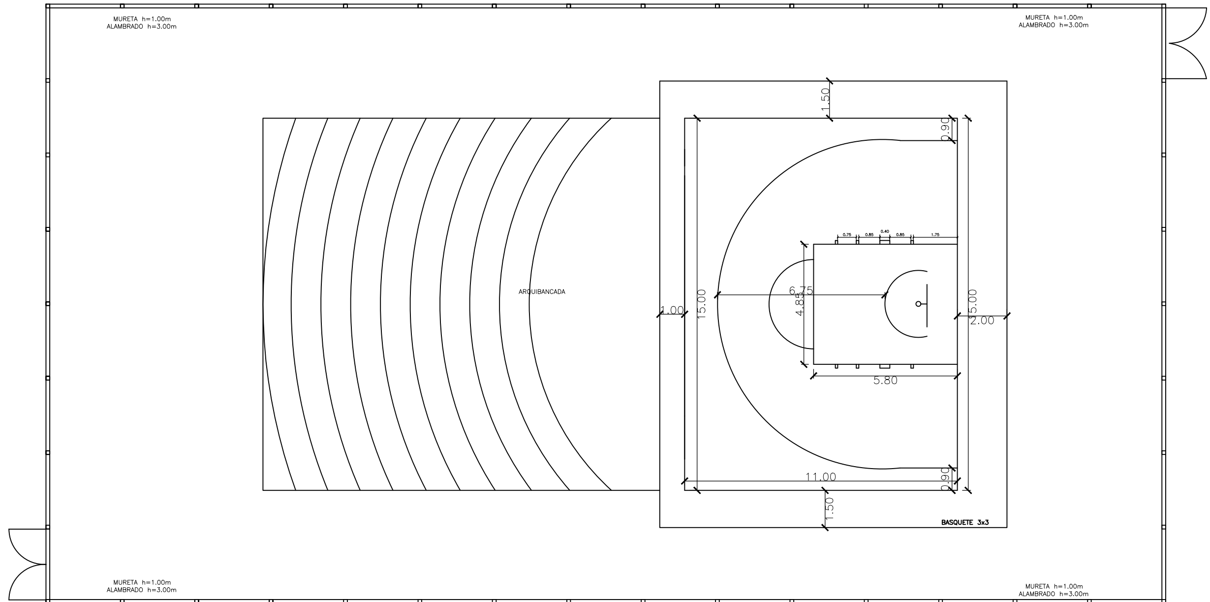
PLANTA-Baixa ESC: 1:150
